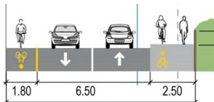
Fig. 2 : Profil au droit du projet VALTRALOC
