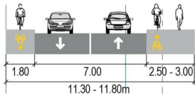
Fig. 1: Profil au droit de la mobilité douce entre Bossonnens et Attalens
