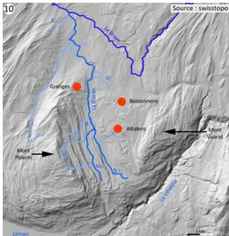
Fig 10 : La Biorde, tracé naturel repris de la carte Siegfried pour la partie méridionale. Ne sont pas figurés les canaux d'assèchement, structures artificielles, ni les nombreuses sources et résurgences du flanc est du mont Pèlerin. Les affluents nommés sont le ruisseau des Barussels (B.), la Goletta (G.), le Corbéron (C.) et le ruisseau des Thioleyres (T.) ; les sous-affluents des derniers cours d'eau ne sont pas dessinés. Autres abréviations : b.i. (bras inférieur) et b.s. (bras supérieur). Les sources d'un cours d'eau peuvent être nombreuses (6 pour la Venoge) et varier selon le critère considéré (altitude, débit, distance depuis une confluence ou une source, géomorphologie, us et coutumes locales...)
